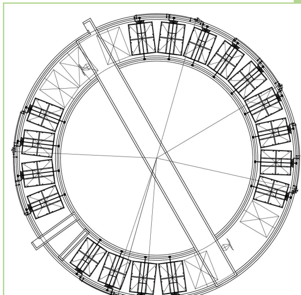
Dessin conforme à l'exécution du bassin
