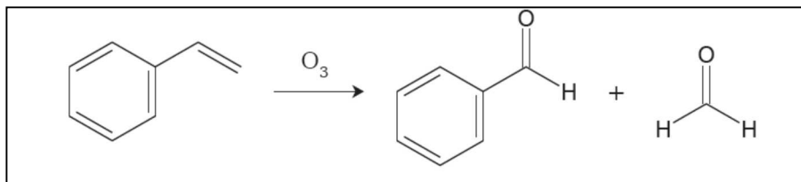
Figuur 2. Partiële oxidatie van styreen via ozon
